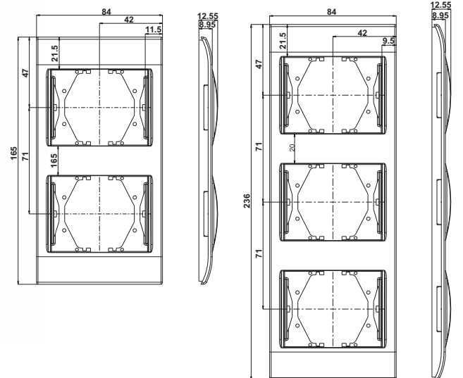
Üçlü Dikey Çerçeve
